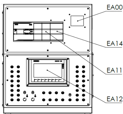
Coffret platine automate EA10 modulable prévu pour recevoir les codes optionnels associés
