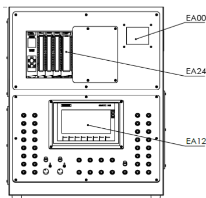
Coffret platine automate EA20 modulaire prévu pour recevoir les codes optionnels associés
