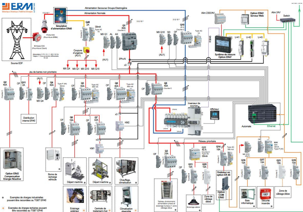
Synoptique TGBT/TGE Communicant Ermadis – Version Industrielle et Tertiaire
