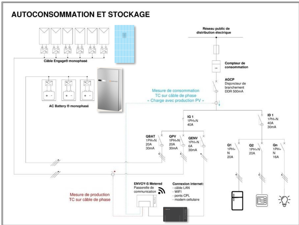
Synoptique d'une installation classique Enphase
