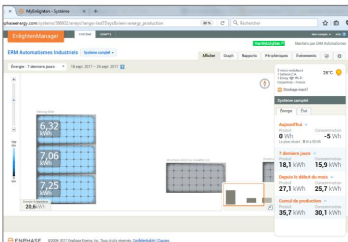
Synoptique d'une installation avec les performances globales
