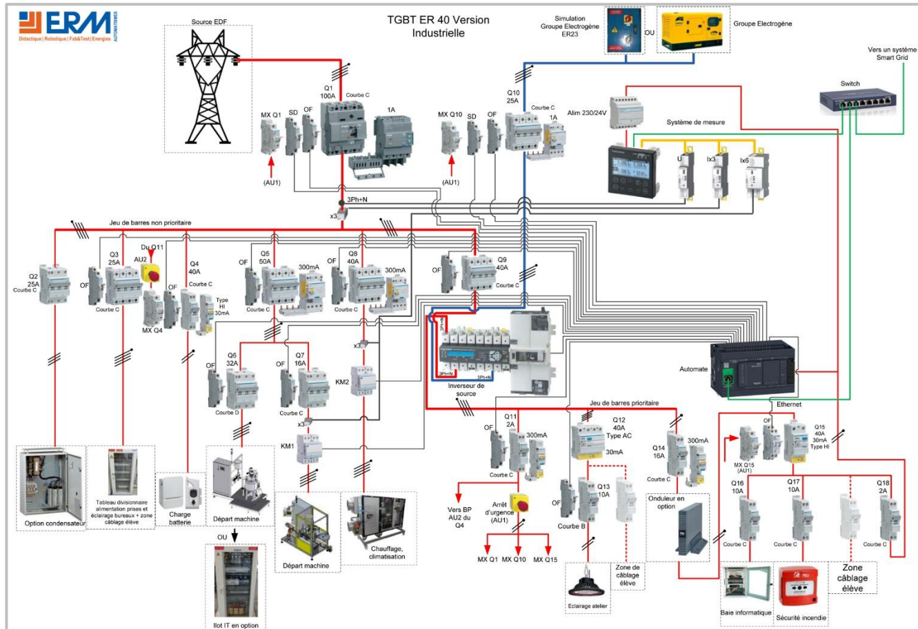
Synoptique TGBT/TGE Communicant Ermadis – Version Industrielle
