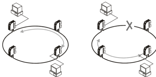
Exemple d'architecture optique en anneau
