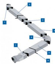
Ensemble de composants pour réseau de raccordement en « faux plafond » avec conduit rectangulaire
