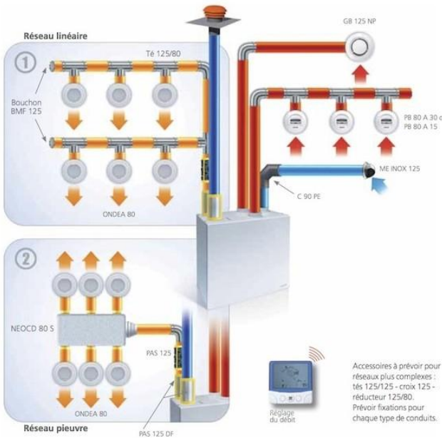
Différentes configurations de réseau aéraulique
