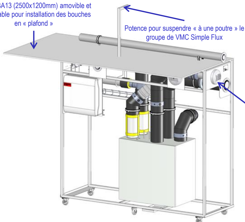
Exemple de mise en œuvre de VMC Double Flux sur le châssis VM12
